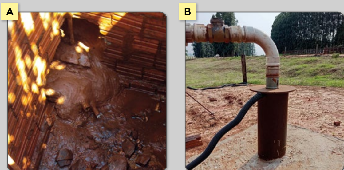
Figura 75 – A) Nascente protegida; B) Poço artesiano-.
