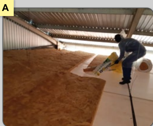
Figura 41 – Lã de vidro sobre a forração do galpão.
