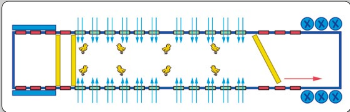
Figura 56 – Ausência de cortina transversal dianteira em aviário com inlet alojado em frente à entrada frontal.
