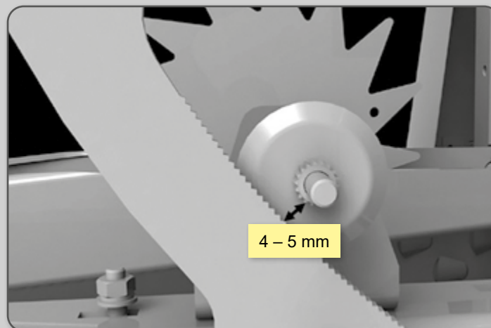
Figura 80 – Distância do acionador do nosador até o rolete.
