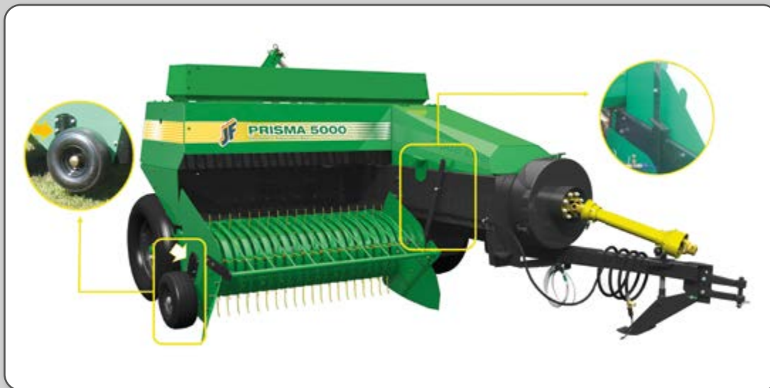
Figura 86 – Rodas para regulagem da altura de recolhimento.
