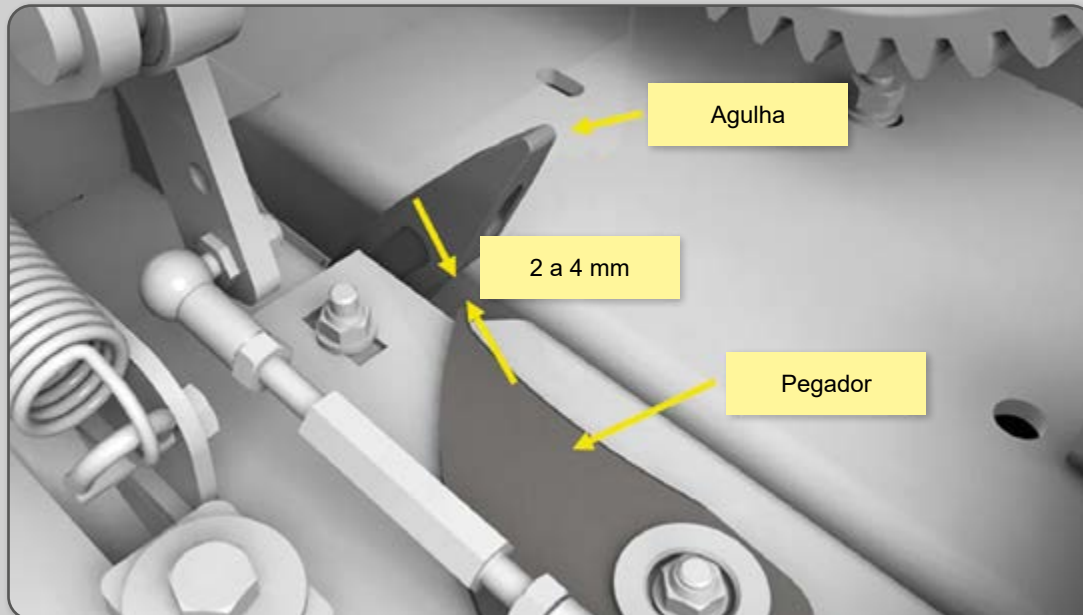
Figura 77 – Distância da agulha ao pegador.
