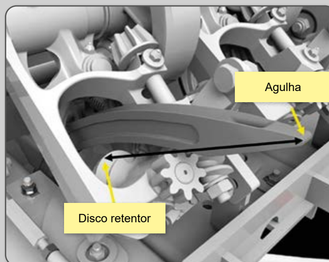
Figura 76 – Distância da agulha ao disco.
