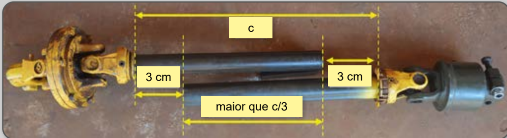
Figura 24 – Sobreposição das partes do eixo cardã.
