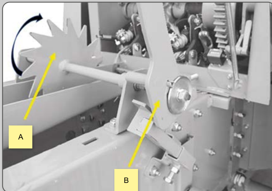
Figura 73 – Regulagem das agulhas com os nosadores.
