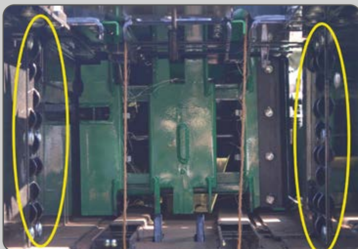
Figura 59 – Placas de retenção.
