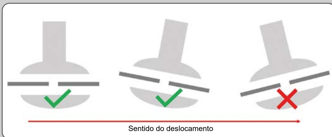
Figura 46 – Regulagem da altura de corte.
