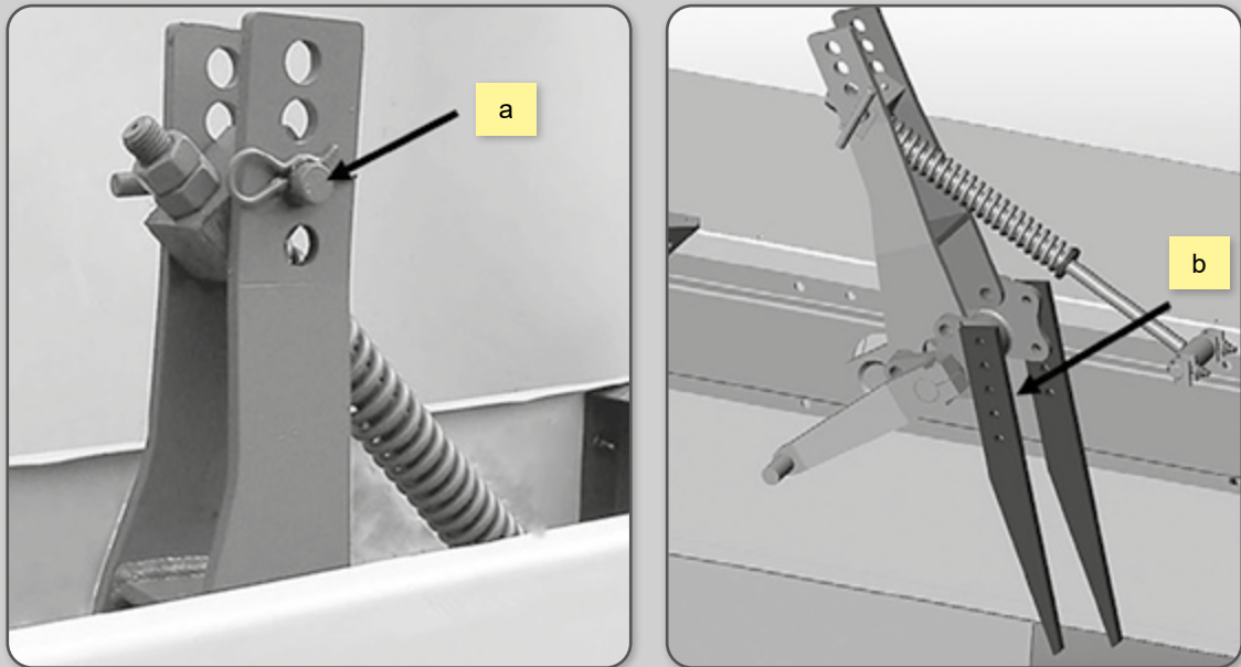
Figura 87 – Regulagem dos garfos de alimentação.
