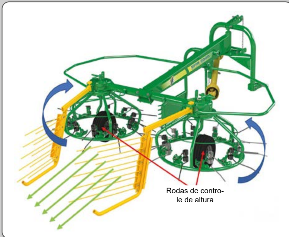
Figura 51 – Rotores girando em sentido oposto, com a forragem saindo no centro, e rodas de controle de altura.
