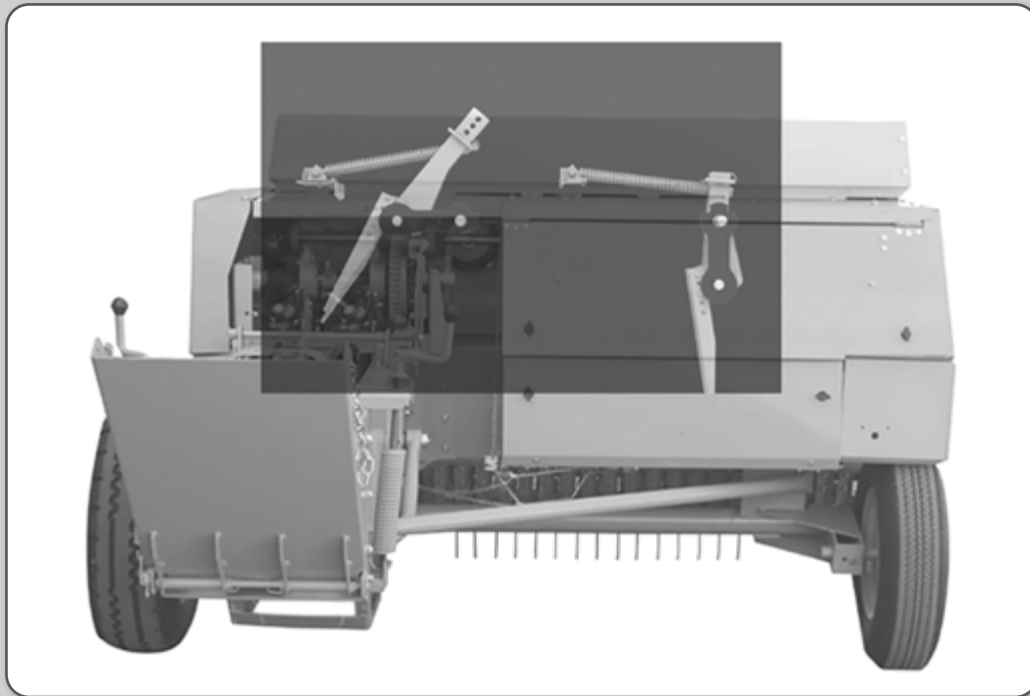
Figura 55 – Mecanismo alimentador composto de garfos.
