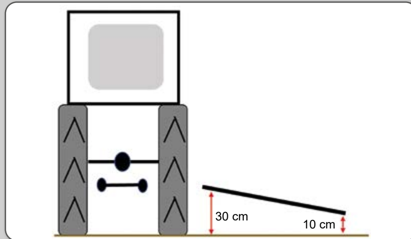
Figura 39 – Regulagem da altura de corte da ceifadora: barra de corte.
