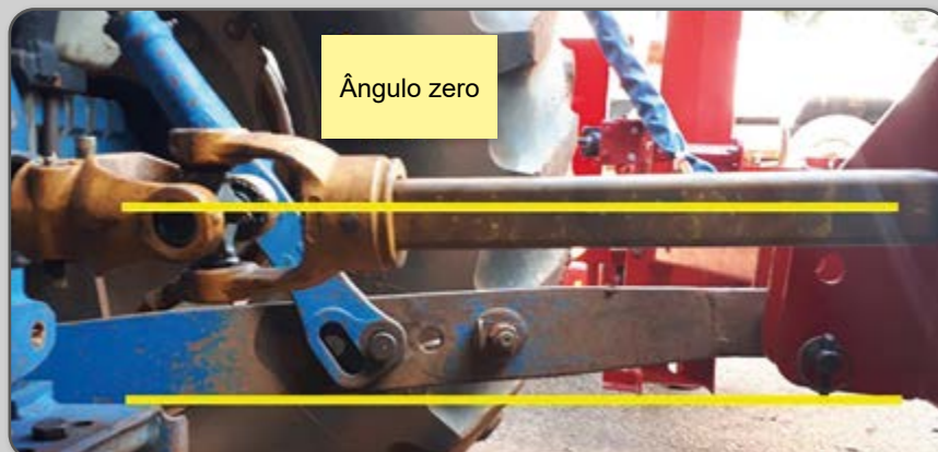
Figura 33 – Eixo cardã na posição ideal.
