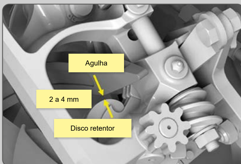
Figura 74 – Regulagem da agulha com o disco retentor.
