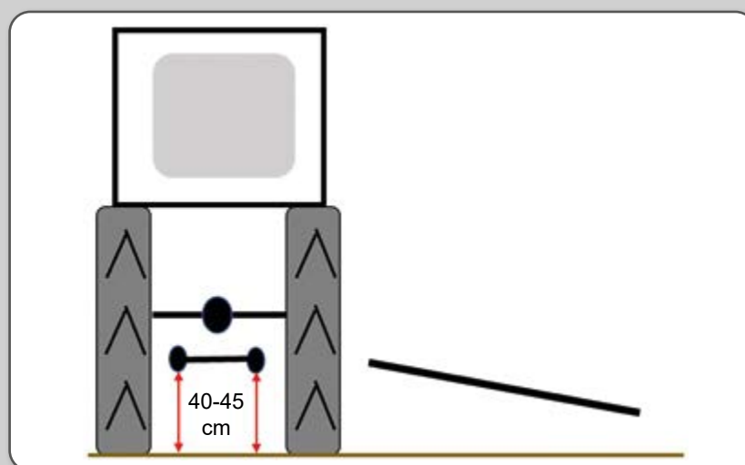
Figura 40 – Regulagem da altura de corte da ceifadora: braços inferiores do sistema hidráulico.
