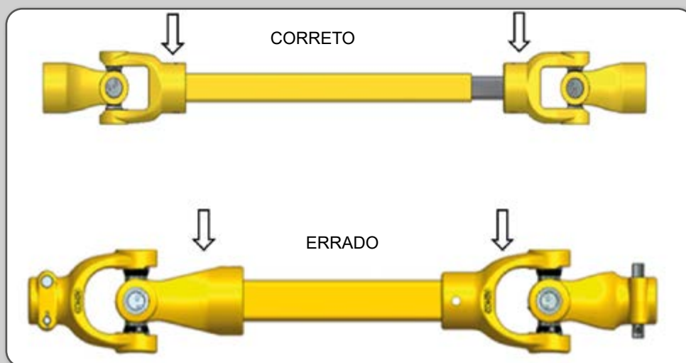
Figura 32 – Montagem correta do eixo cardã.
