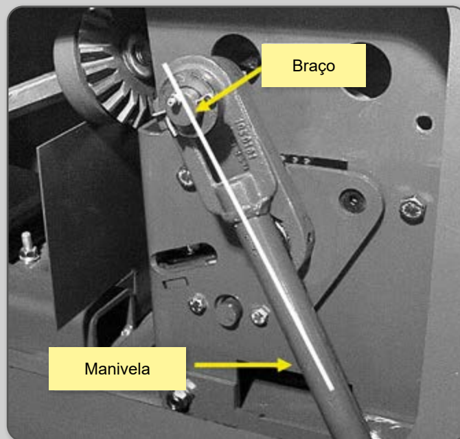
Figura 75 – Regulagem do avanço das agulhas.
