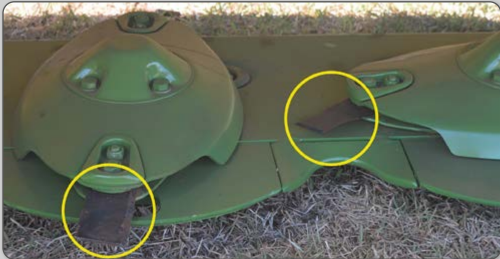
Figura 19 – Facas.
