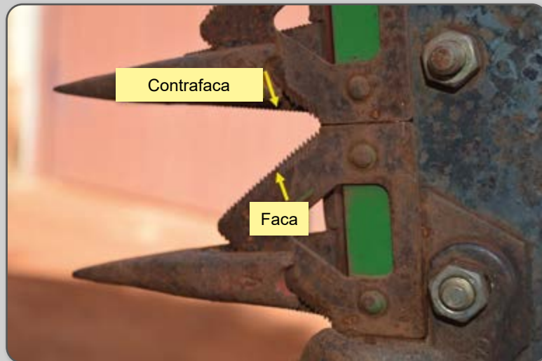
Figura 6 – Faca oscilatória e contrafaca.
