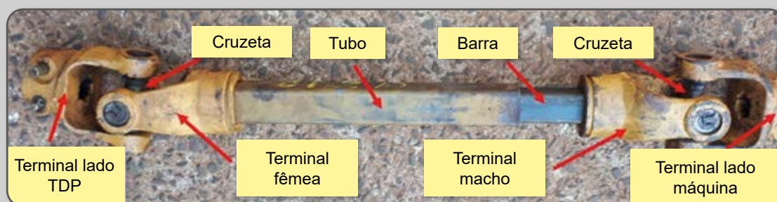
Figura 21 – Partes do eixo cardã.
