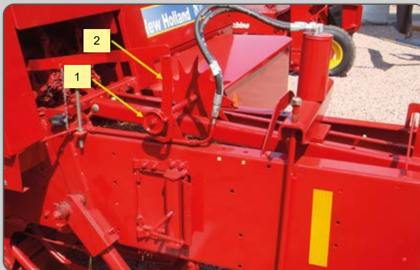
Figura 88 – 1) Polia do mecanismo de amarração e 2) Braço disparador do atador-nosador.
