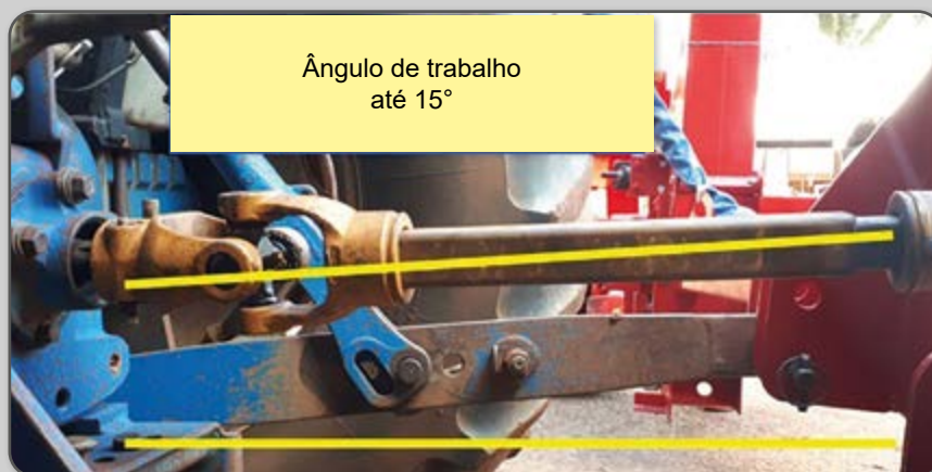
Figura 34 – Eixo cardã na posição ideal em até 15°.
