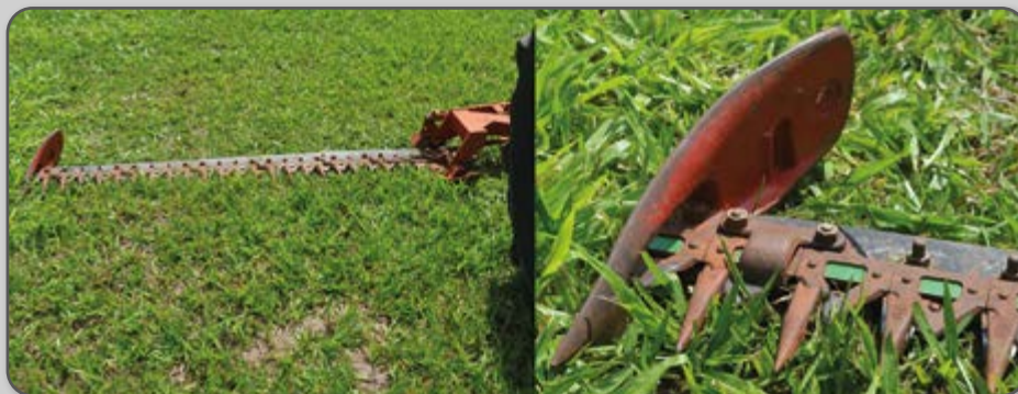
Figura 5 – Defletor localizado no patim externo da barra de corte.
