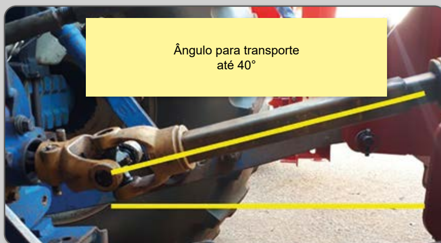
Figura 35 – Eixo cardã na posição ideal em até 40° para transporte.
