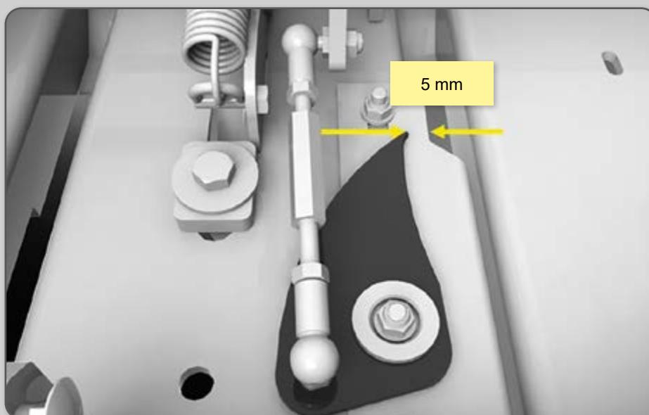
Figura 78 – Distância do pegador.
