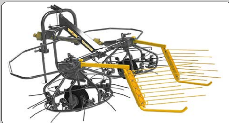
Figura 48 – Ancinho rotativo de dupla função: enleirador e espalhador.
