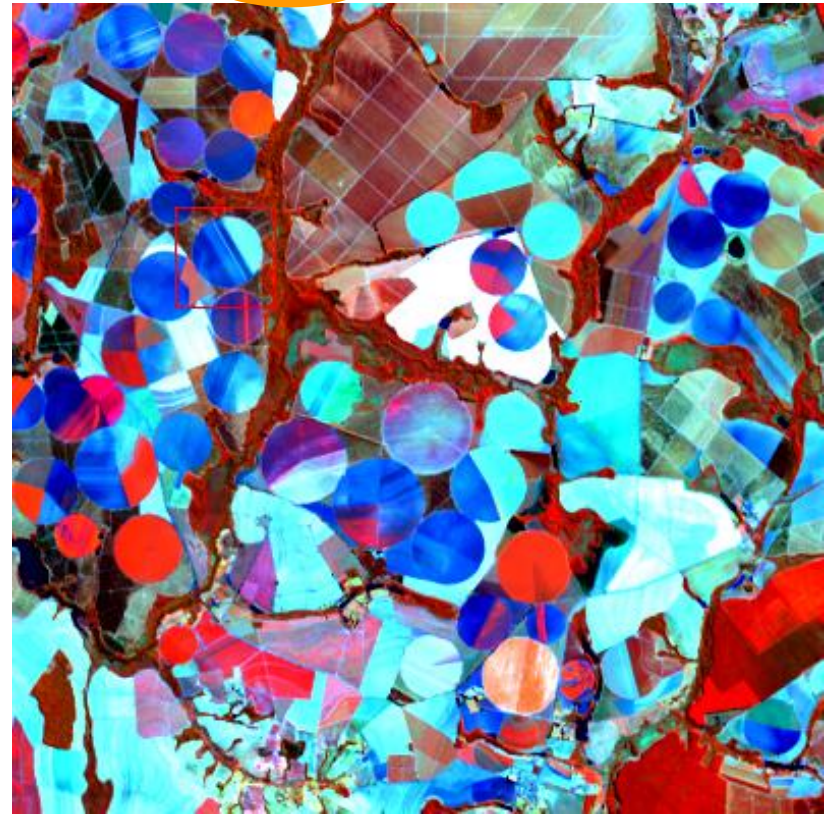
Landsat-8/OLI-08
